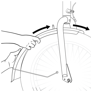
Voer het spatbord vanaf de achterkant van het voorwiel door
