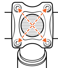
Draai de bouten vast in een "X"-patroon
