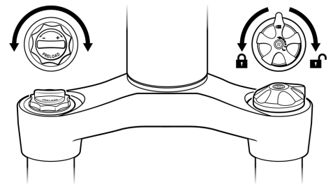
Stoßdämpfergabel
