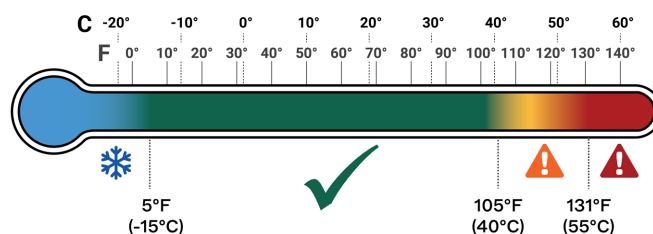
BETRIEB: Empfohlener Temperaturbereich
