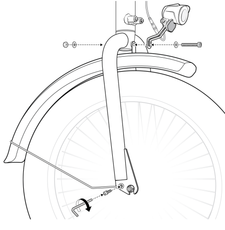
Matériel de montage du phare et du garde-boue
