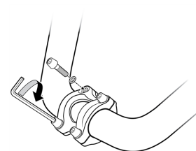
Boulons de plaque frontale de potence
