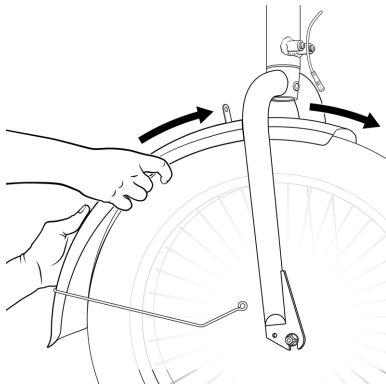
Passez le garde-boue par l'arrière de la roue avant
