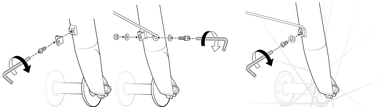
Montage van L-beugel (vereist op sommige fietsen)
