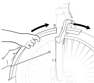
Voer het spatbord vanaf de achterkant van het voorwiel door
