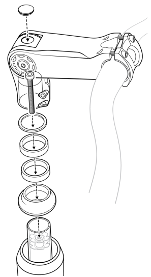
Stuurpen en onderdelen balhoofdagerpers
