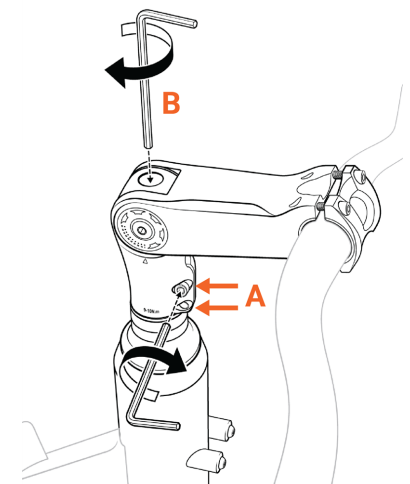
Draai de balhoofdagerpers zorgvuldig strak
