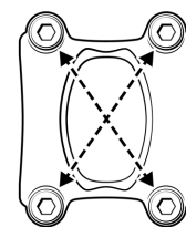
Draai de bouten vast in een "X"-patroon
