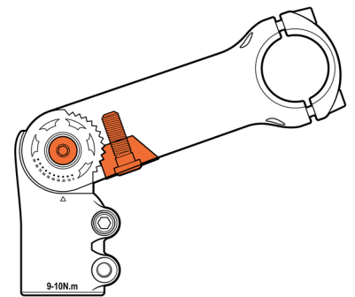
Bouten voor het afstellen van de hoek van de stuurpen (zijkant en onderkant, in oranje)
