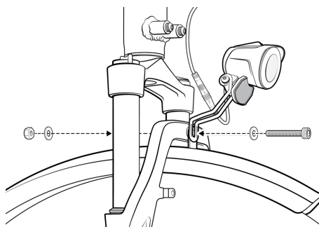
Bevestigingsmateriaal voor voorlicht
